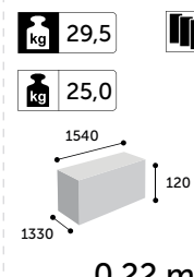
VL2,5 HW / VL2,5 VW + VL W2,5
