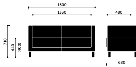
VL2,5 H / VL2,5 V
