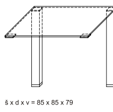
Postavení jednacího stolu PRJS 85 S2
