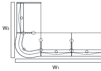
LUV05L + 2xLUV03 02 + LUV04 + LUV03 02 + LUV05P+3xNL41
