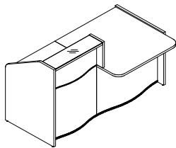
A: LUV05L + LUV03 02 + LUV07P + LUV01 + LUV06P+NL41 B: LUV06L + LUV01 + LUV07L + LUV03 02 + LUV05P+NL41
