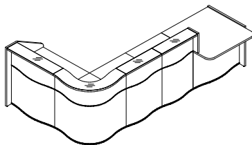
A: LUV06L + LUV01 + LUV07L + 2xLUV03 02 + LUV04 + LUV03 02 + LUV05P+4xNL41 B: LUV05L + LUV03 02 + LUV04 + 2xLUV03 02 + LUV07P + LUV01 + LUV06P+4xNL41
