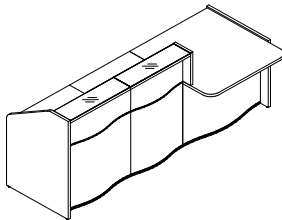
A: LUV05L + 2xLUV03 02 + LUV07P + LUV01 + LUV06P+2xNL41 B: LUV06L + LUV01 + LUV07L + 2xLUV03 02 + LUV05P+2xNL41
