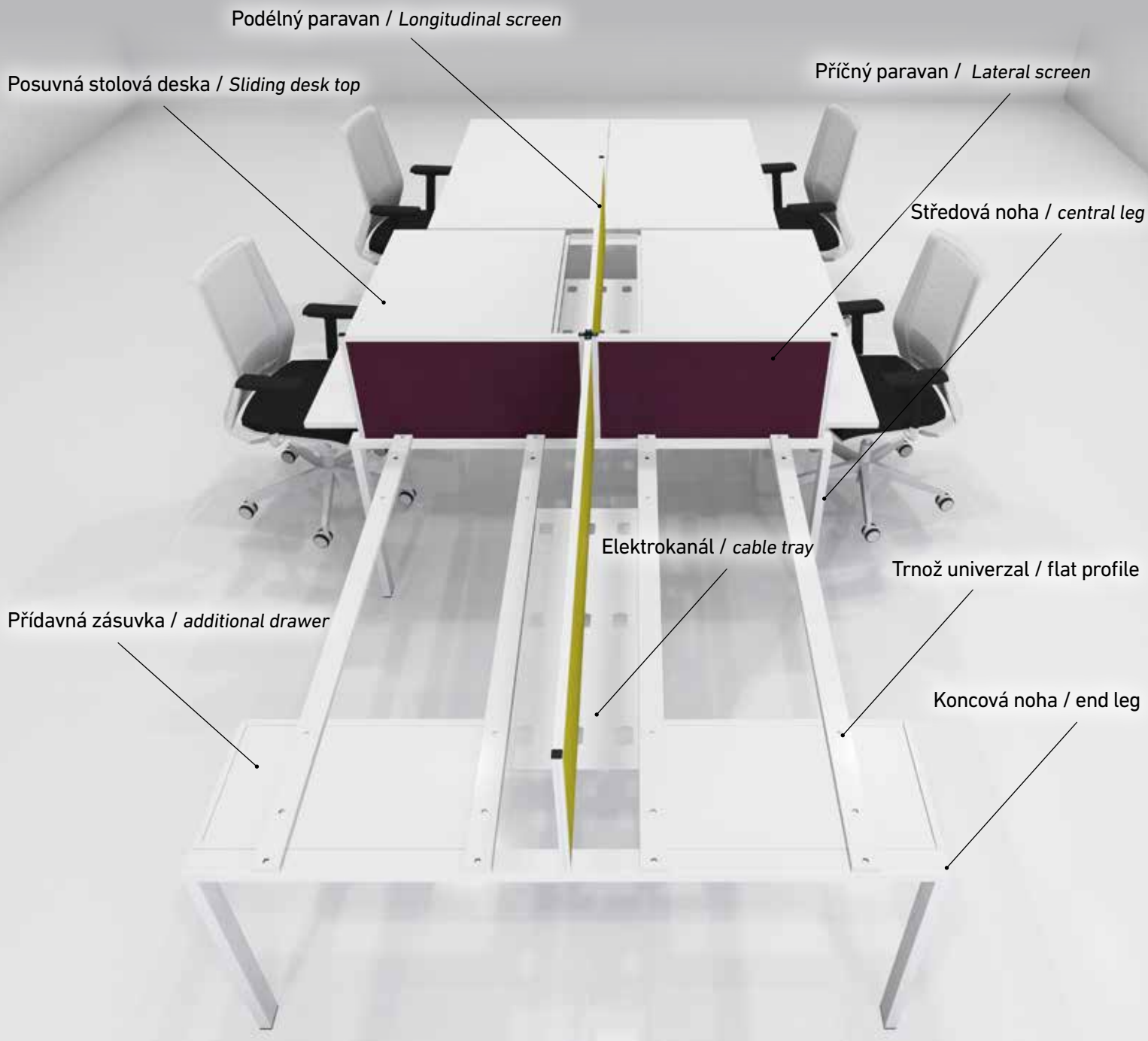
Typové označení stolové sestavy: MUKS160S3 / Type specification of the desk set: MUKS160S3
